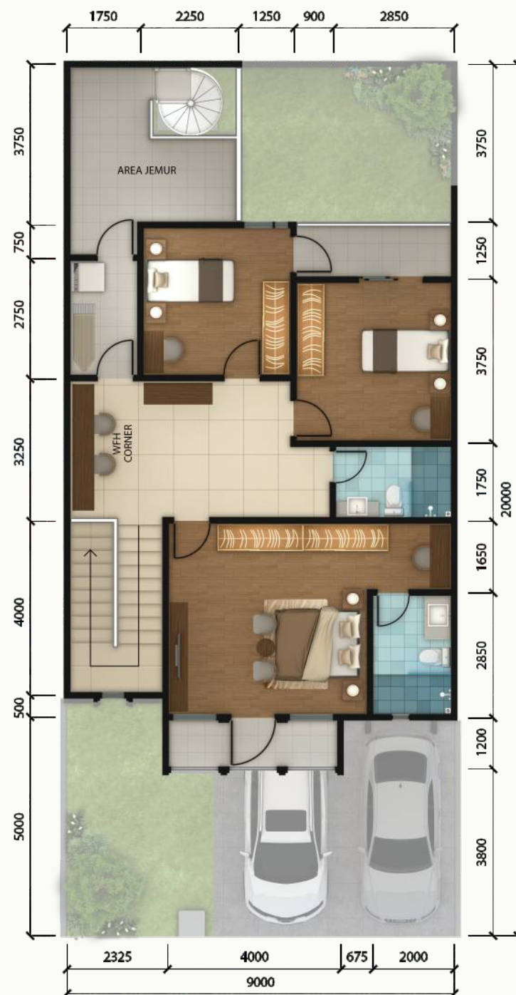
LANTAI ATAS
