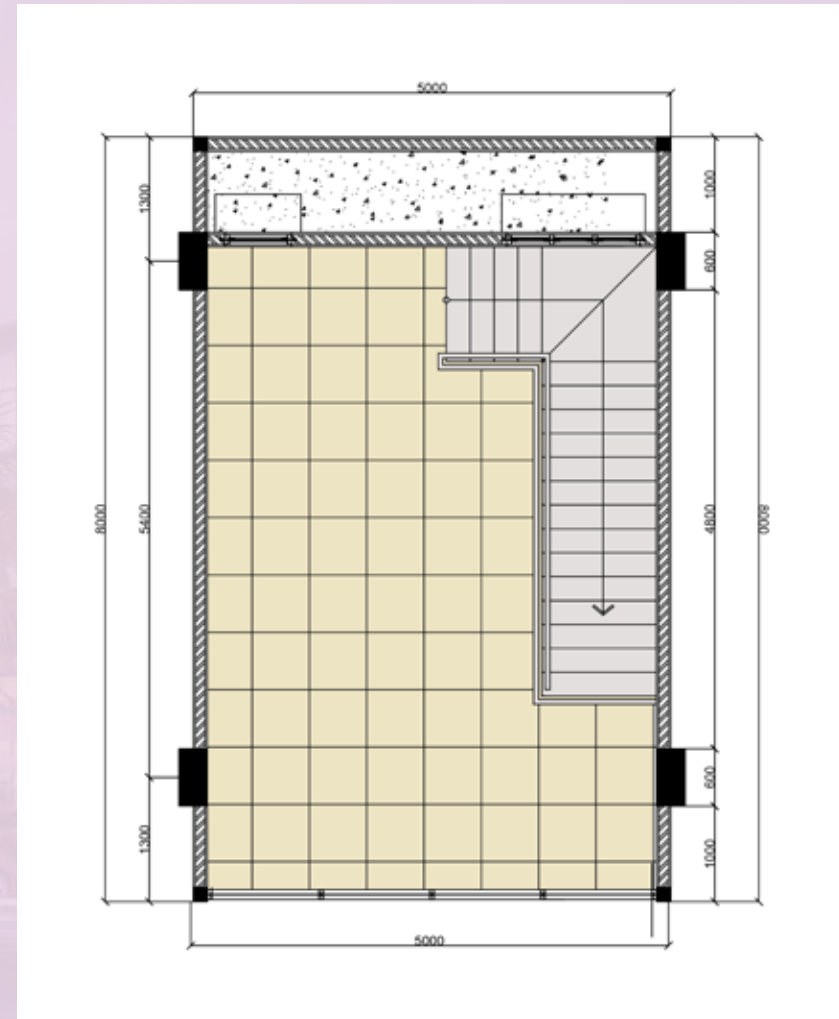
Lantai 2
